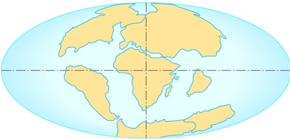
La Terre, il y a 60 millions d'années
