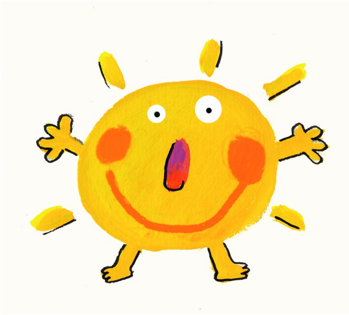
la lune
