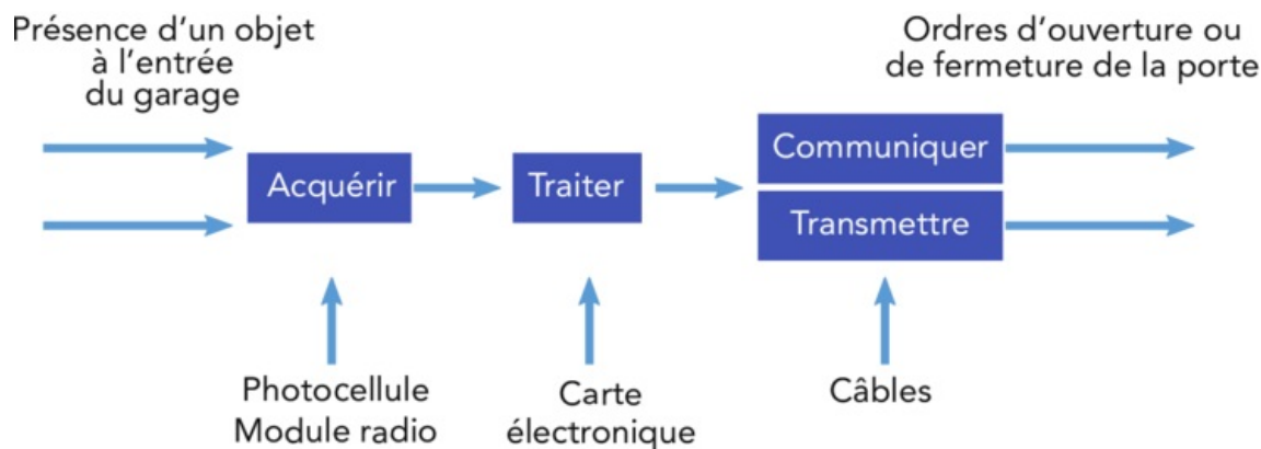
Chaîne d'information d'une porte de garage automatisée
